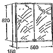
Spegelskåp 560 mm
