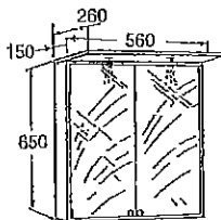
Spegelskåp med halogenramp 560 mm
