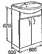
Kommodpaket 600
